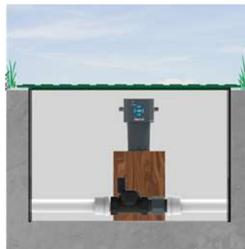
התקנה בתוך ארגז מגופים
